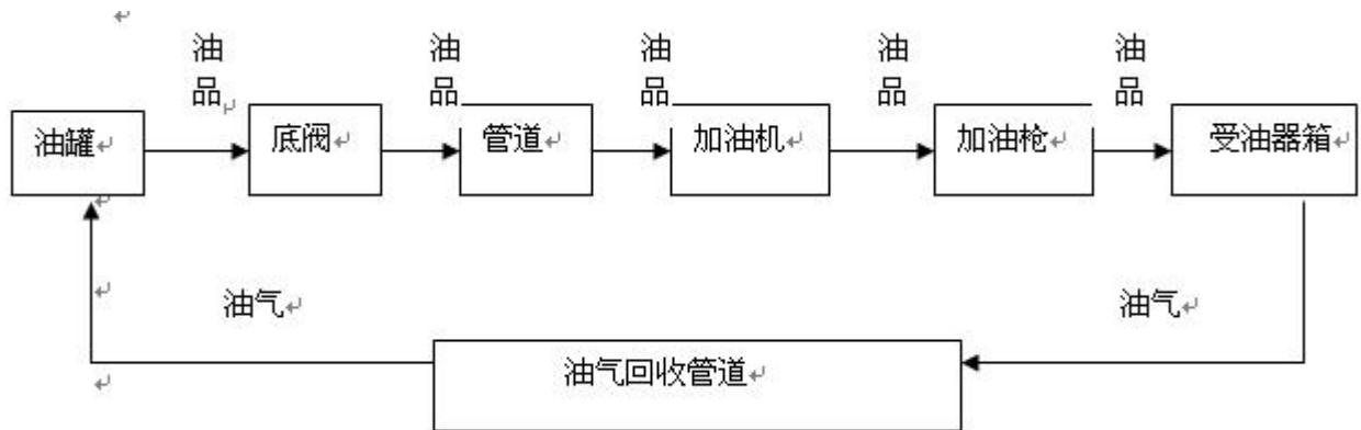
图 2-3 加油工艺流程简图
