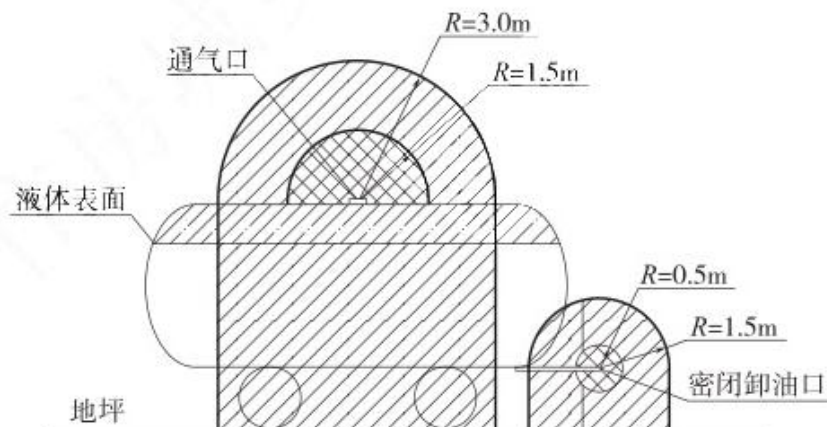
图 C.0.4 汽油油罐车的爆炸危险区域划分
